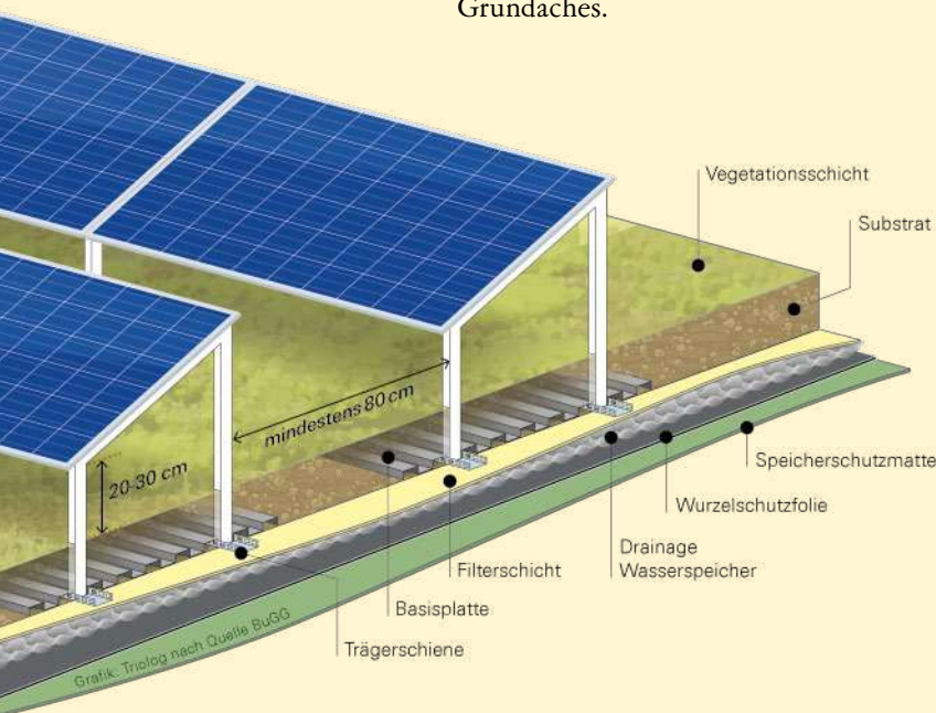
Exemplarischer Aufbau einer Kombination aus Dachbegrünung und Photovoltaik
